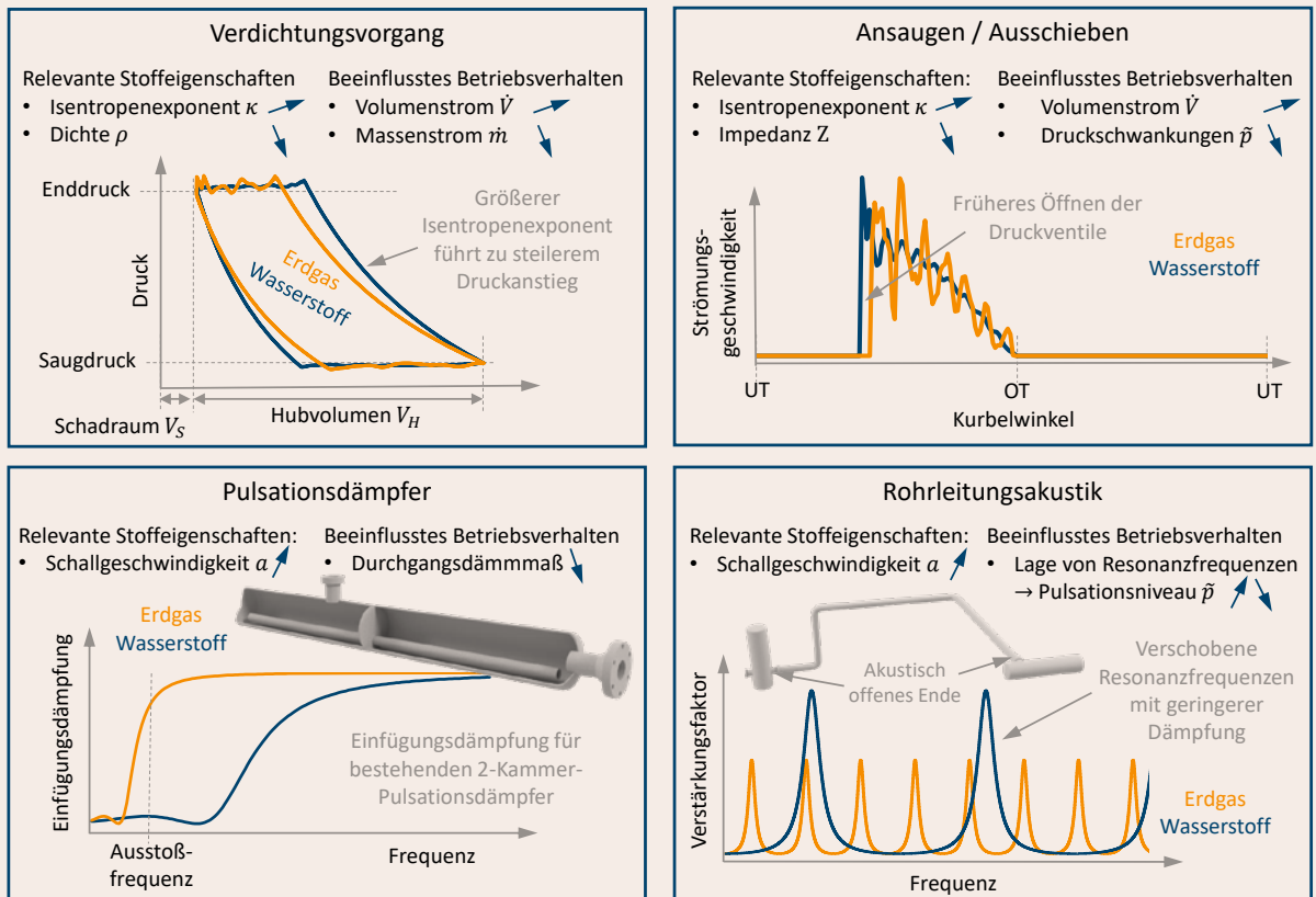
Bild 4: Einfluss von Wasserstoff auf das Pulsationsverhalten von Kolbenverdichteranlagen
