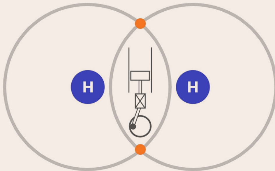
Bild 2: Verdichtung von Wasserstoff mit Kolbenverdichtern
